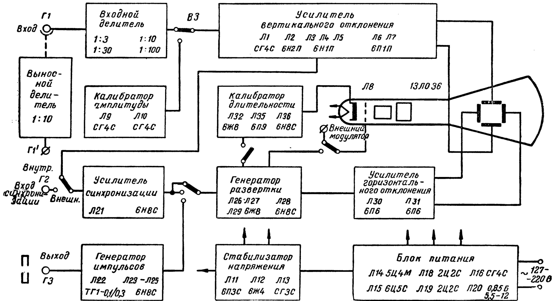
Блок-схема электронного осциллографа
