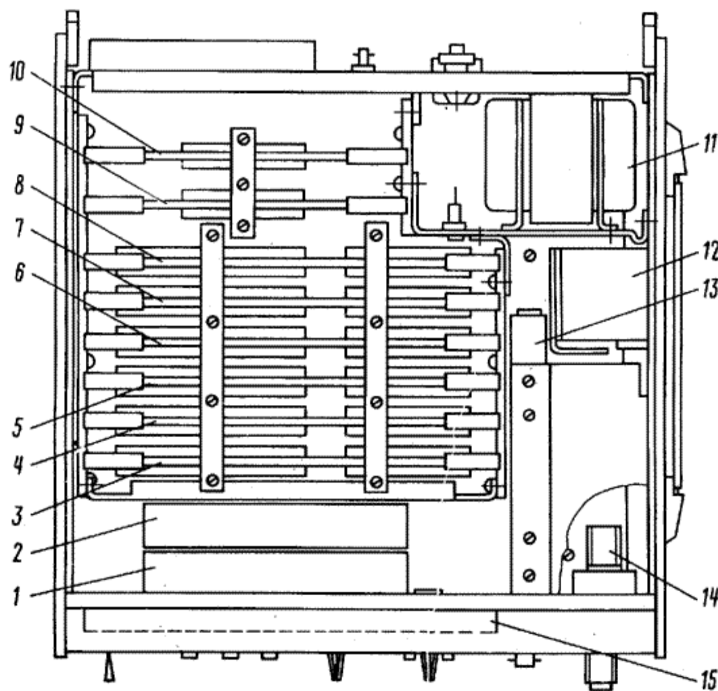
Рис. 1. Размещение основных составных частей: 1 — усилитель ВЧ 2.030.055; 2 — гетеродин 2.205.017 (ЧЗ-68); 2.205.017-1 (ЧЗ-69); 3 — усилитель постоянного тока 2.032.027; 4 — счетчик 3.056.034; 5 — блок управления 3.057.093; 6 — устройство вычислительное управляющее 3.035.033; 7 — устройство запоминающее оперативное 3.065.067; 8 — устройство запоминающее программируемое 3.065.066; 9 — блок стабилизаторов напряжения 3.233.119; 10 — блок стабилизаторов напряжения 3.233.120; 11 — трансформатор 4.700.049; 12 — генератор кварцевый 3.261.006; 13 — усилитель 2.030.052 (ЧЗ-68); 14 — смеситель 2.245.013; 15 — блок индикации 3.045.033 (ЧЗ-68), 3.045.033-01 (ЧЗ-69)
