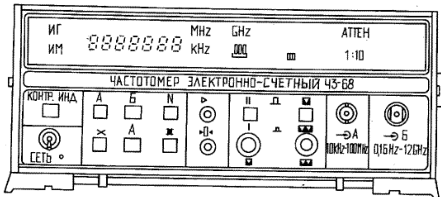
Рис. 1. Частотомер ЧЗ-68
