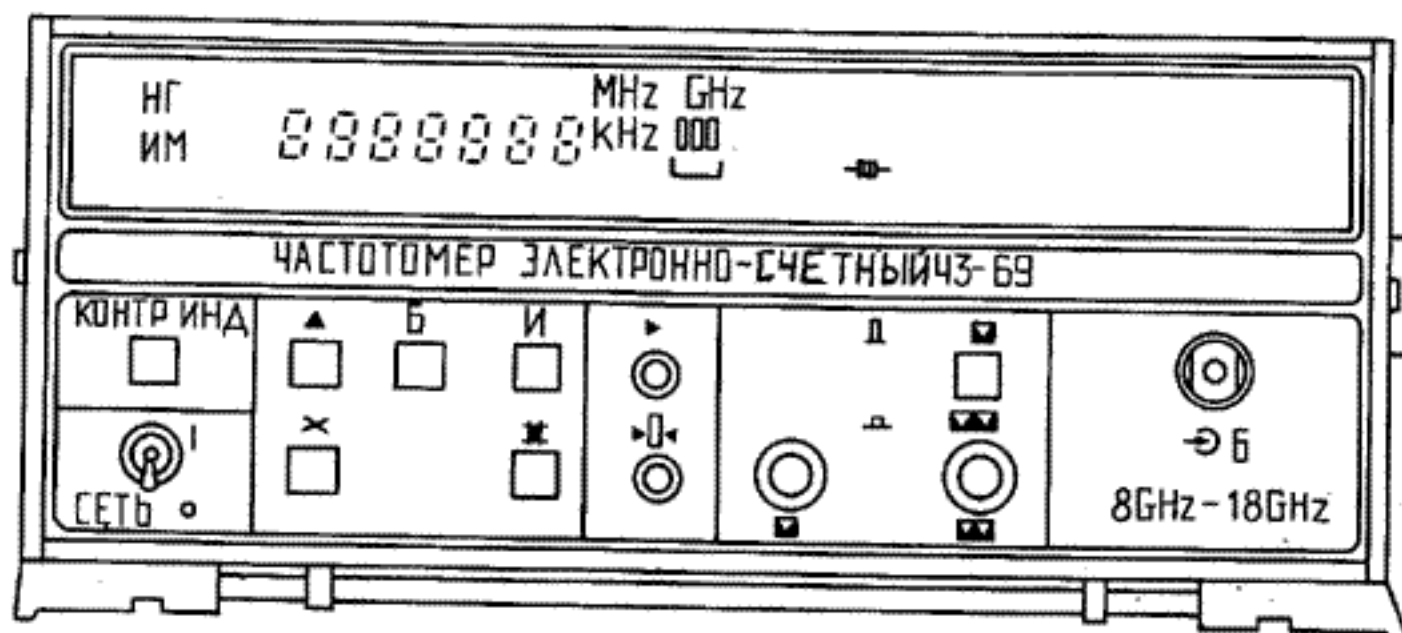
Рис. 2. Частотомер ЧЗ-69
