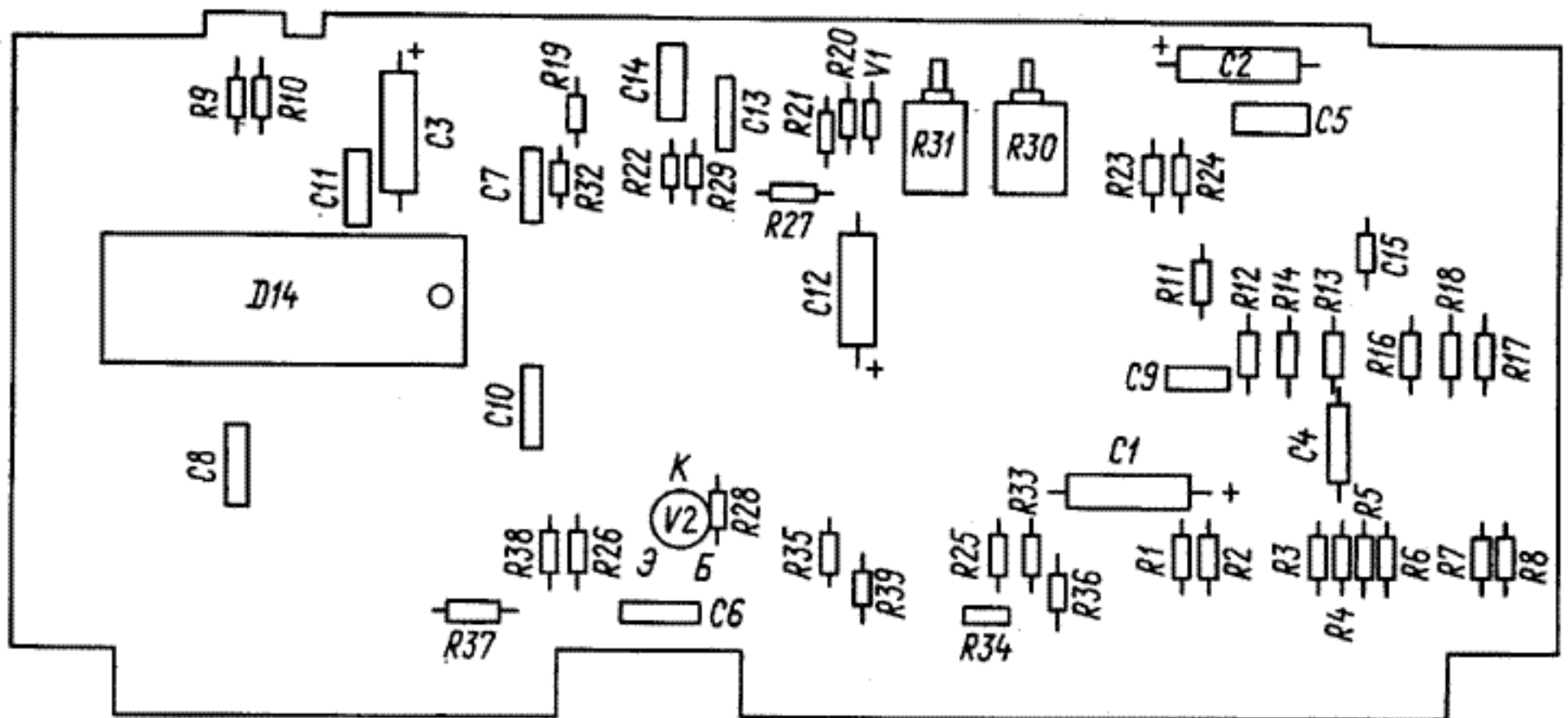
Рис. 7. Устройства вычислительное управляющее 3.035.033 (вид со стороны монтажа)
