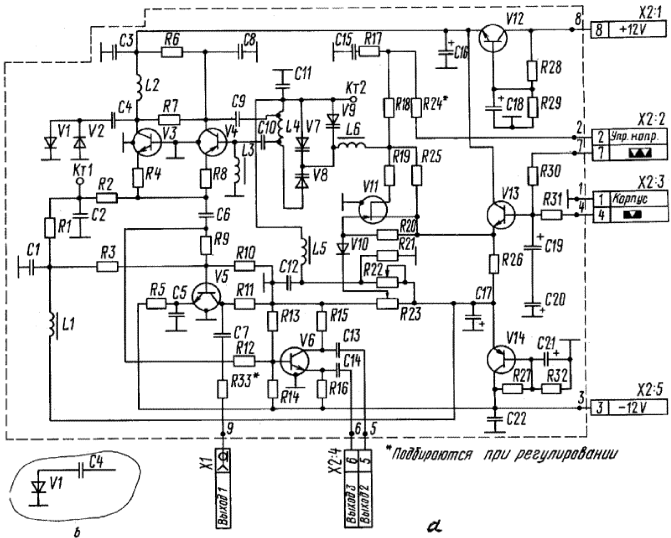
Рис. 4. Схема электрическая принципиальная гетеродина: а - 2.205.017; б - 2.205.017-01
