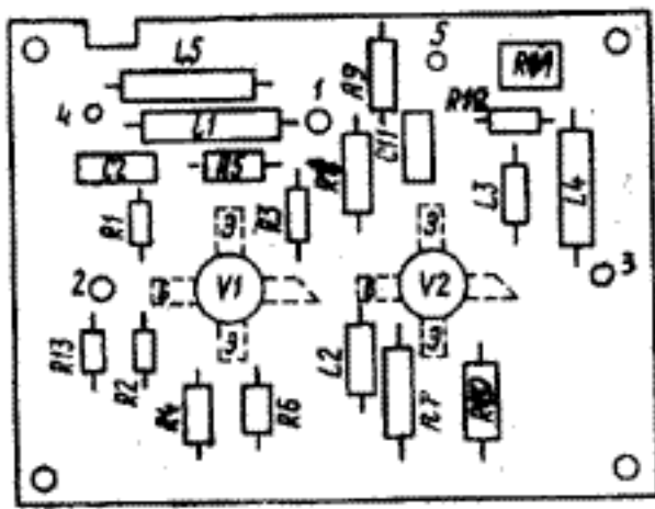
Рис. 3. Усилитель ВЧ 2.030.066
