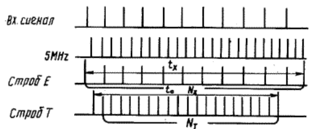
Рис. 3. Формирование измеряемого интервала времени
