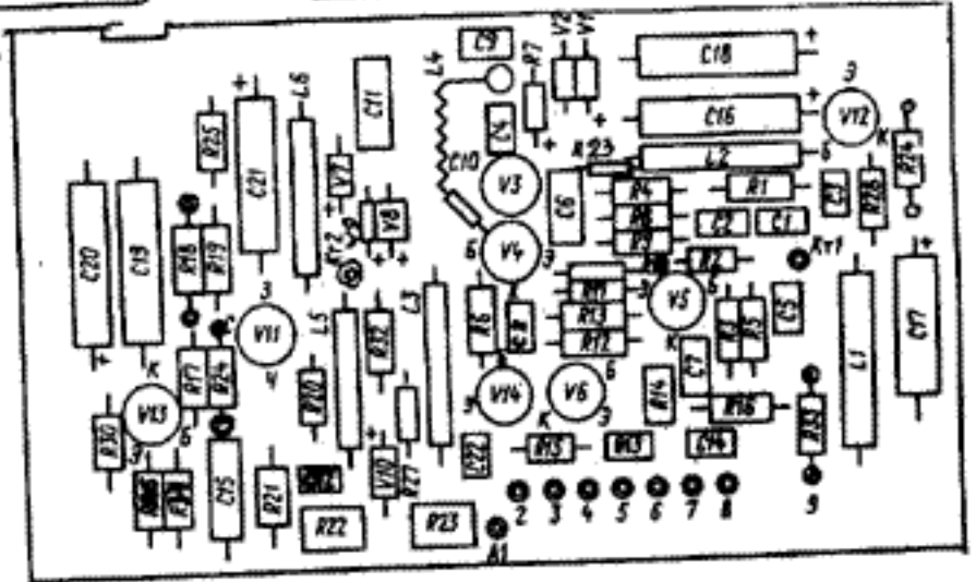
Рис. 6. Гетеродин 2.205.017
