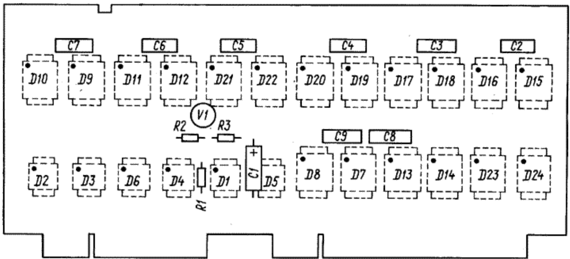
Рис. 16. Устройство запоминающее оперативное 3.065.067
