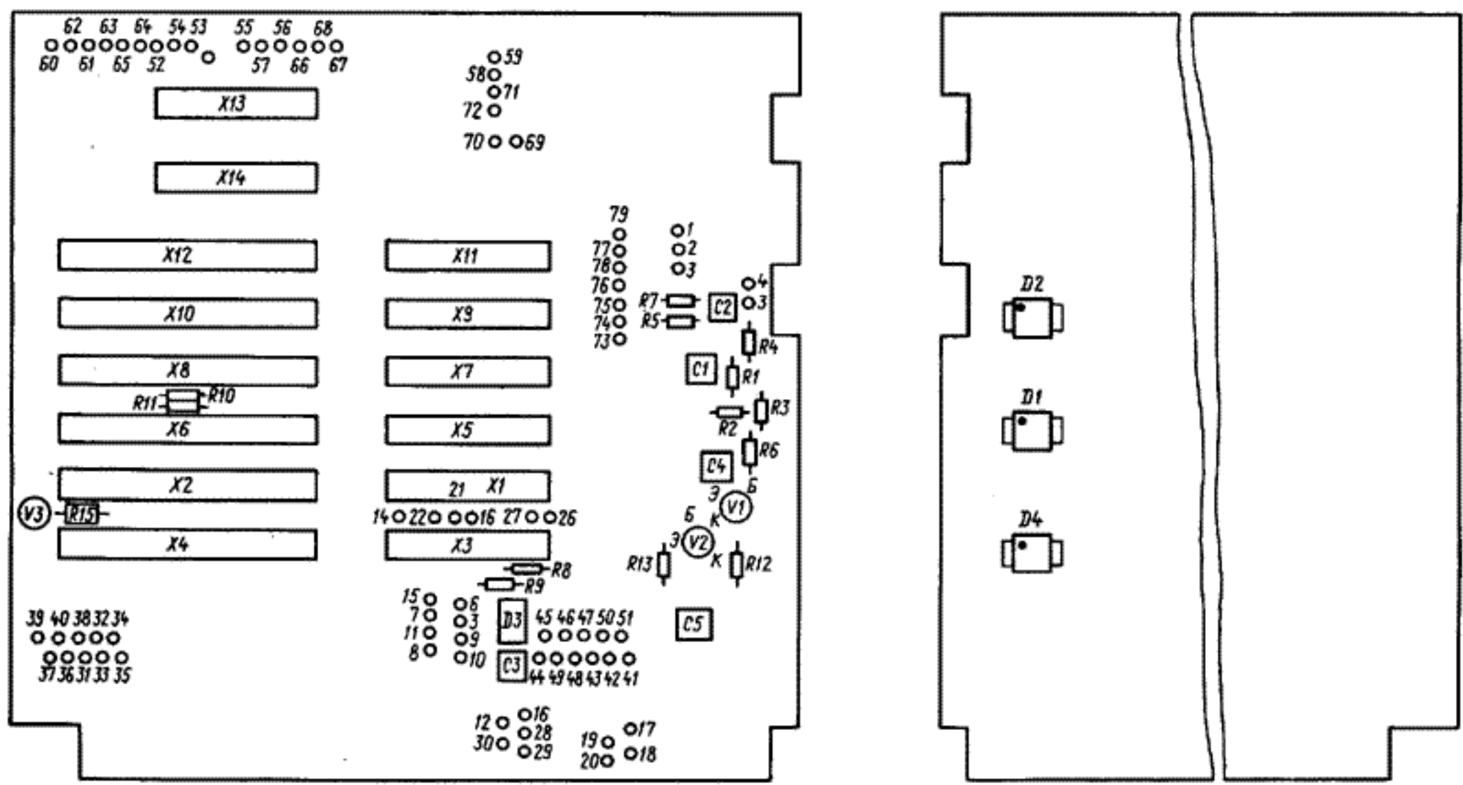
Рис. 20. Частотомер 5.171.007
