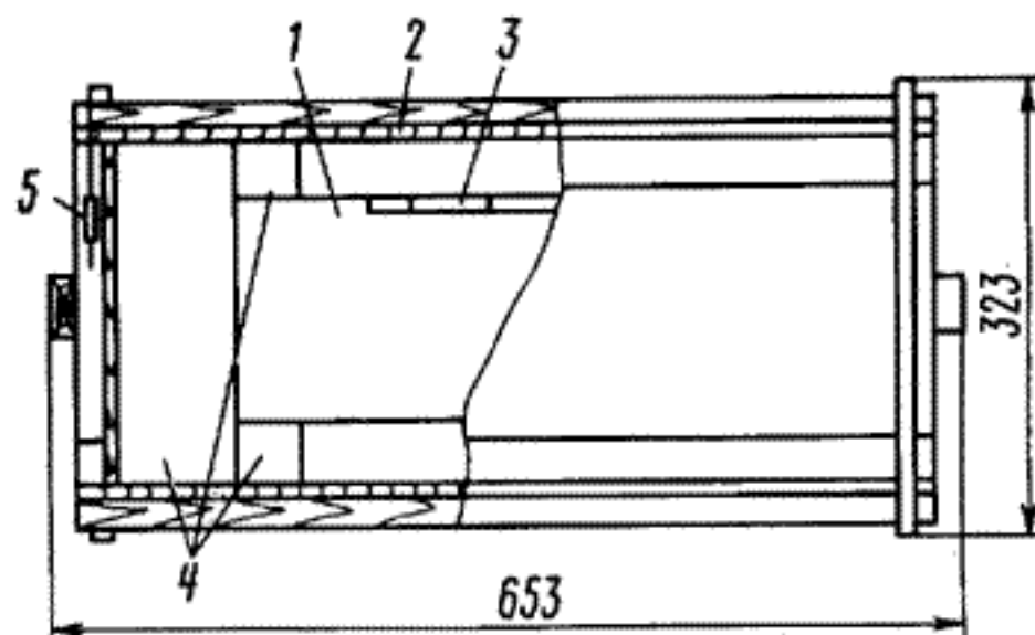
Рис. 9. Схема упаковки:
