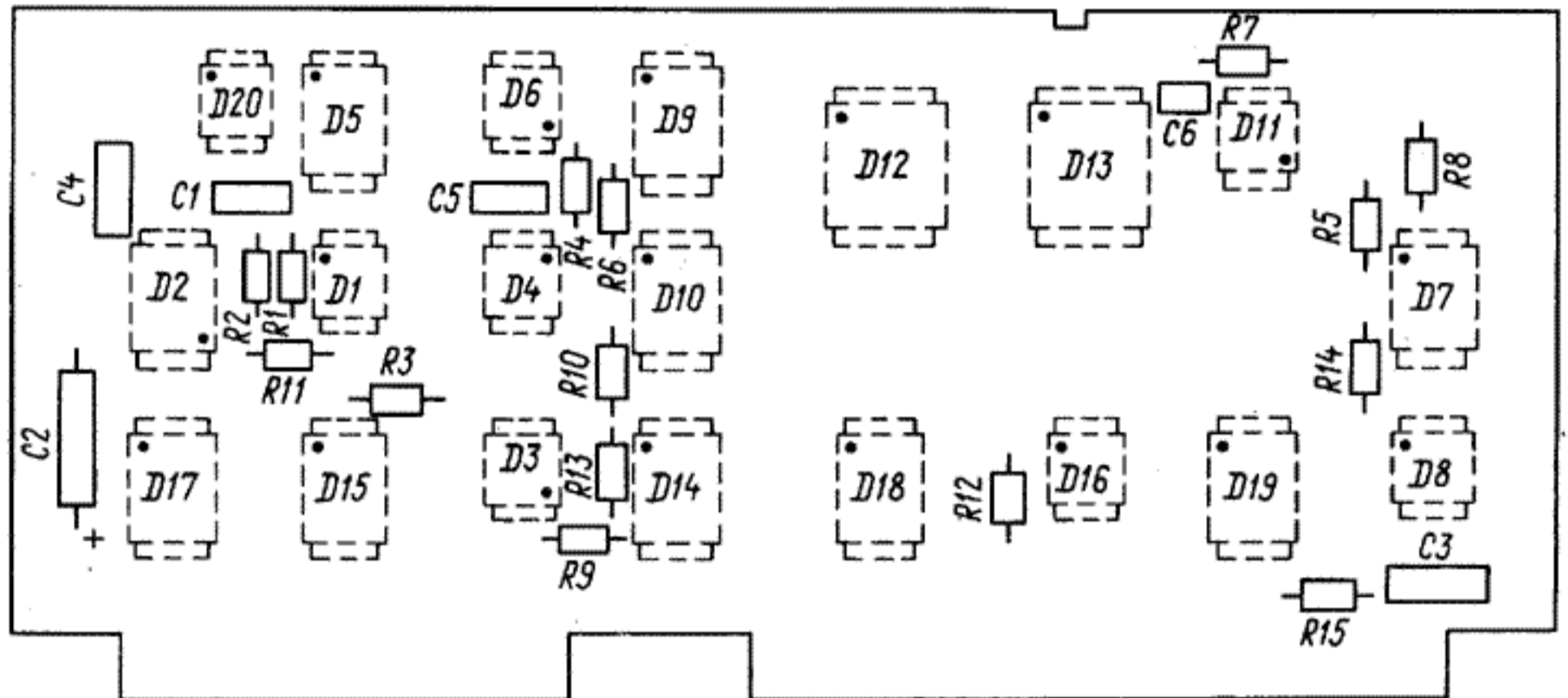
Рис. 13. Блок управления 3.057.093
