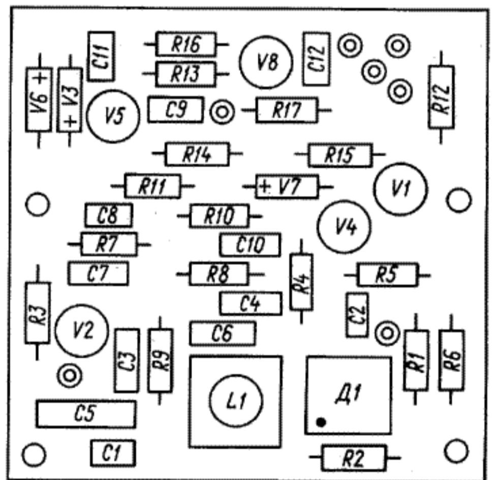
Рис. 19. Генератор кварцевый 3.261.006
