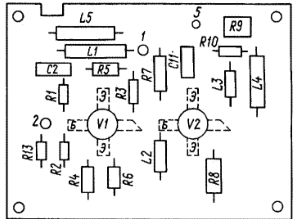
Рис. 3. Усилитель ВЧ 2.030.055
