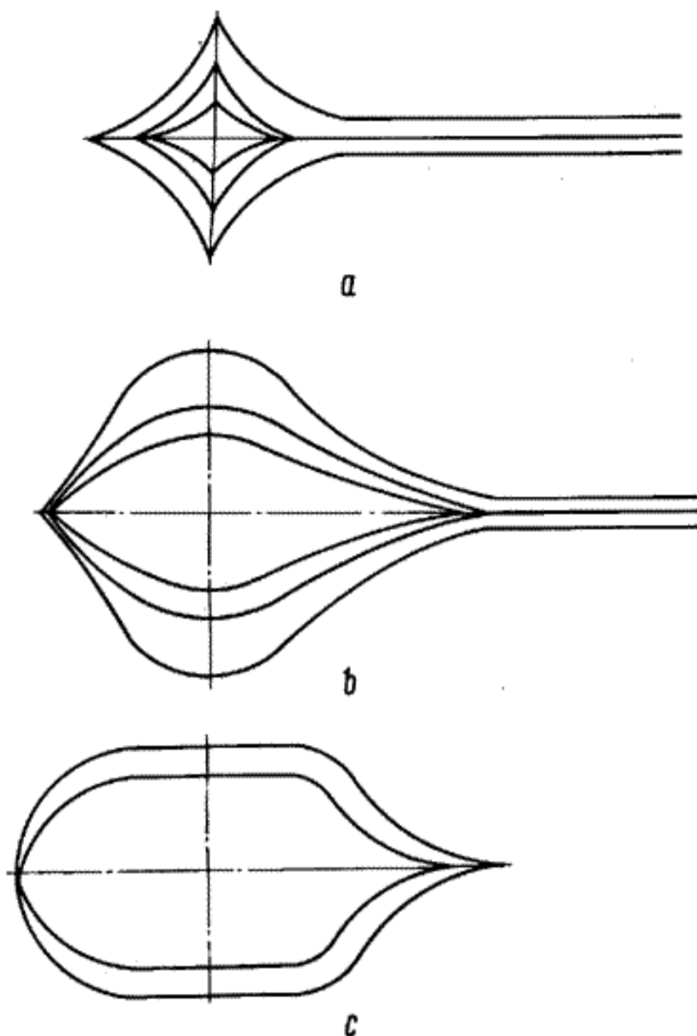
Рис. 7. Осциллограммы нулевых биений: а — длительность 0,3 мкс, период — 3,3 кГц, переключатели осциллографа в положении: V/ДЕЛ — 0,5, ВРЕМЯ/ДЕЛ — 1 мкс; б — длительность — 1 мкс, период 1 кГц, переключатели осциллографа в положении: V/ДЕЛ — 1, ВРЕМЯ/ДЕЛ — 2 мкс; с — длительность — 10 мкс, период 100 Гц, переключатели осциллографа в положении: V/ДЕЛ — 2, ВРЕМЯ/ДЕЛ — 10 мкс
