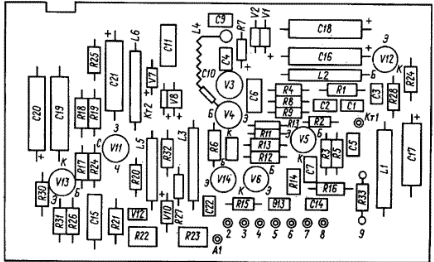
Рис. 6. Гетеродин 2.205.017
