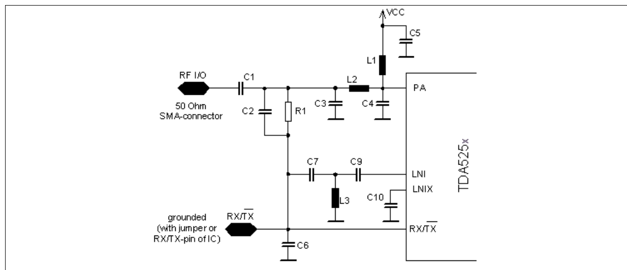
TX_Mode.wmf
