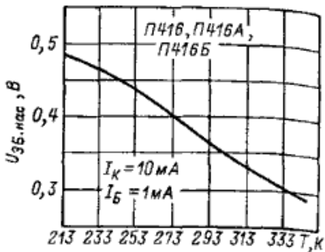
Зависимость напряжения насыщения эмиттер-база от температуры.
