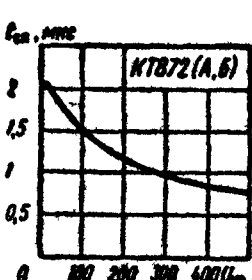
Зависимость времени спада от напряжения коллектор — эмиттер
