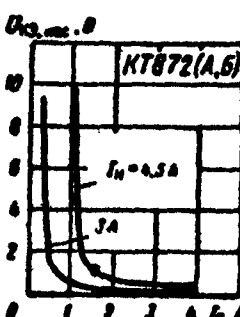
Зависимости напряже- ния насыщения коллек- тор — эмиттер от тока базы
