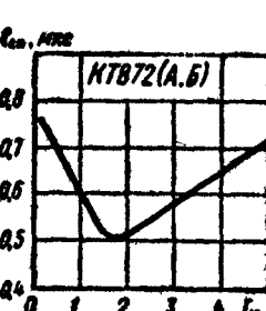
Зависимость времени спада от тока коллек- тора
