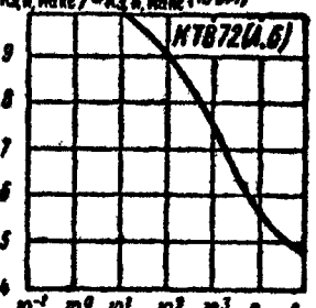
Зависимость максимал- но допустимого им- пульсного напряжения коллектор — эмиттер от сопротивления база — эмиттер
