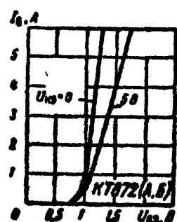
Входные характеристики
