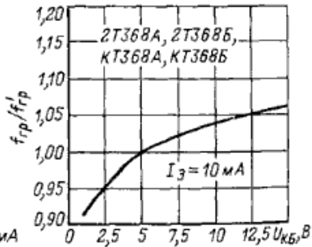
Зависимость относительной граничной частоты от напряжения коллектор-база
