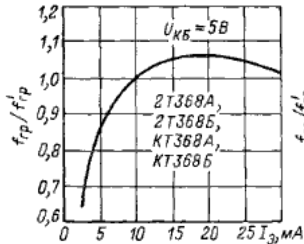
Зависимость относительной граничной частоты от тока эмиттера
