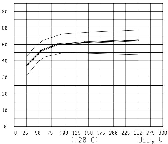
I_{del}(ON) , мкА
