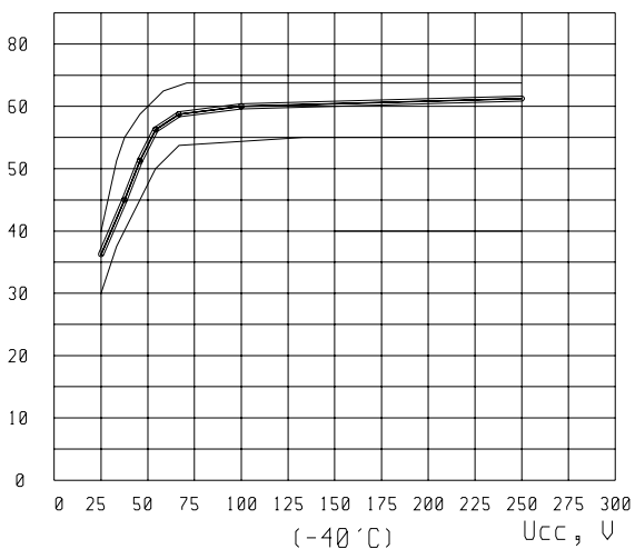
I_{del}(ON) , мкА
