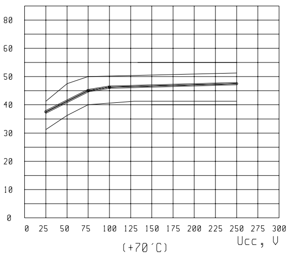
I_{del}(ON) , мкА
