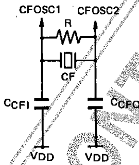
Fig. 13 CF oscillation
